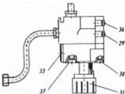
Zawór gazowy EUROGAS PL 12, EUROGAS PL 16, EUROGAS PL 20
