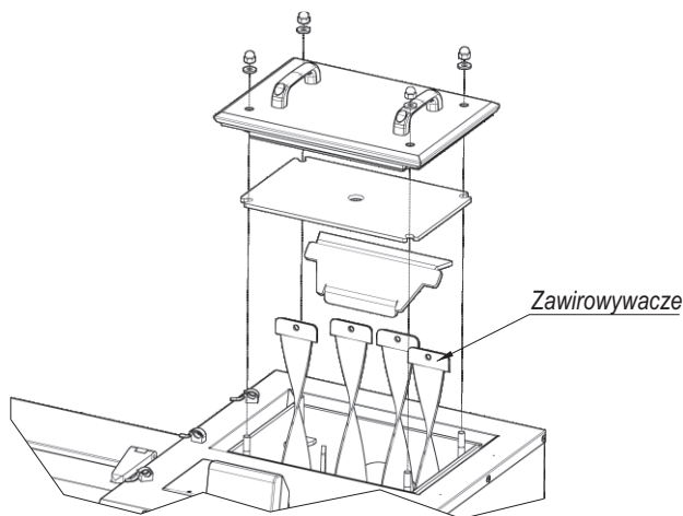
Rysunek 16. Sposób czyszczenia zawiorowycze.
