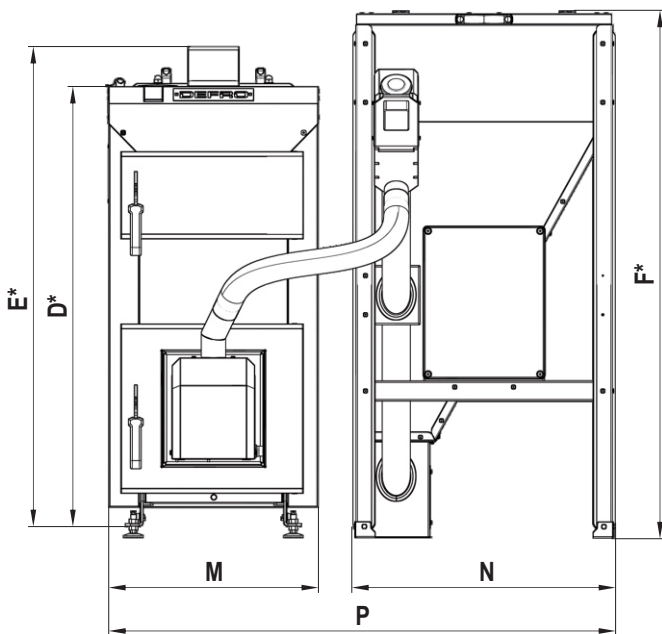
Rysunek 1. Podstawowe wymiary kotłów.
