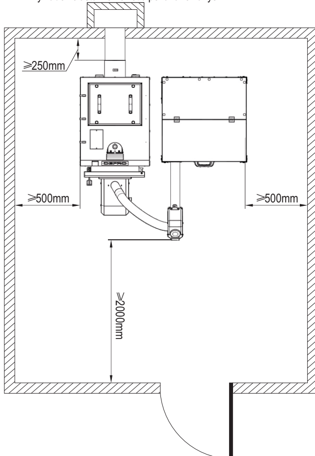
Rysunek 4. Ustawienie kotła w pomieszczeniu kotłowni.
