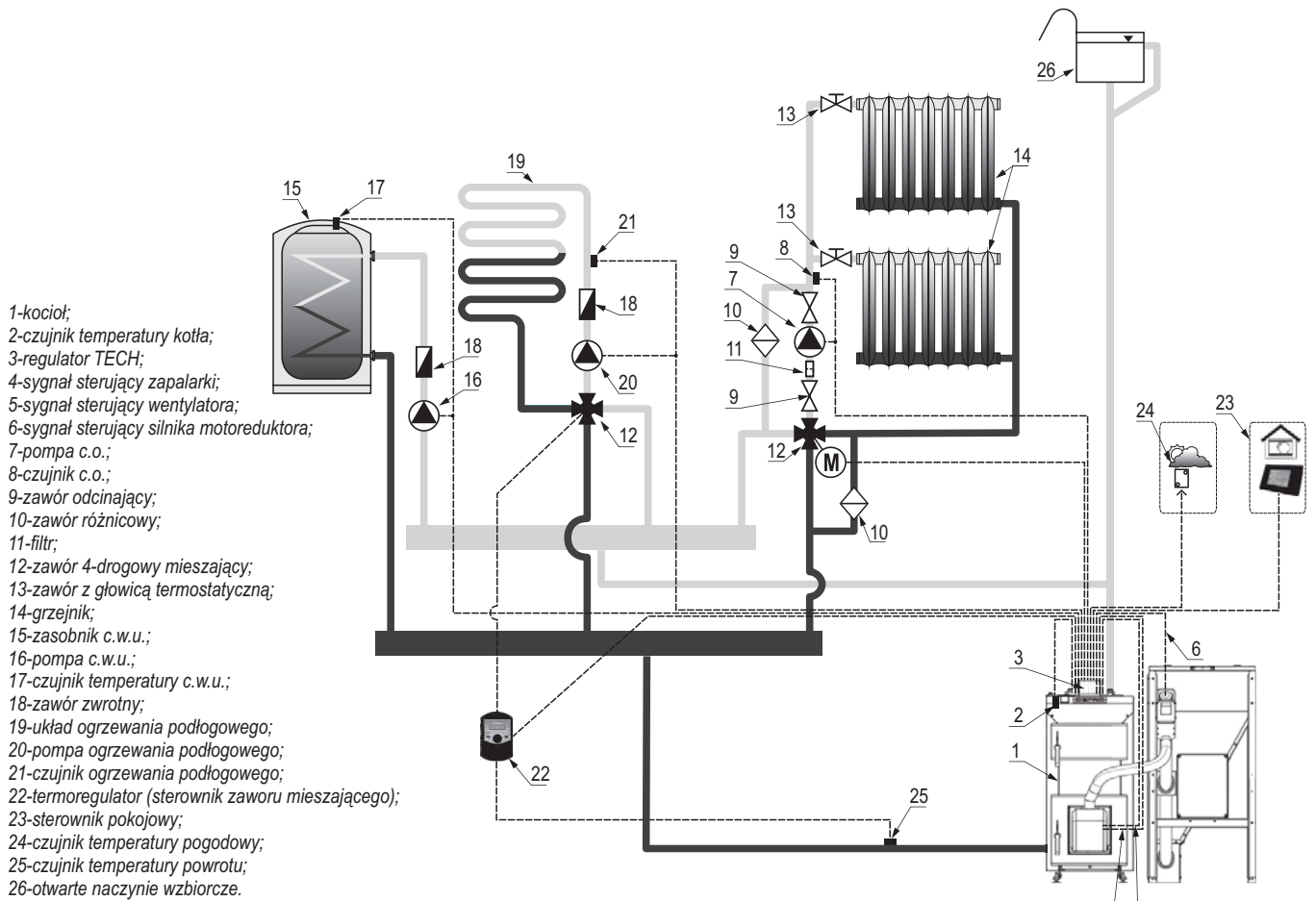
Rysunek 12. Przykładowy schemat instalacji grzewczej systemu otwartego z ochroną temperaturą kotła realizowaną przez termoregulator.
