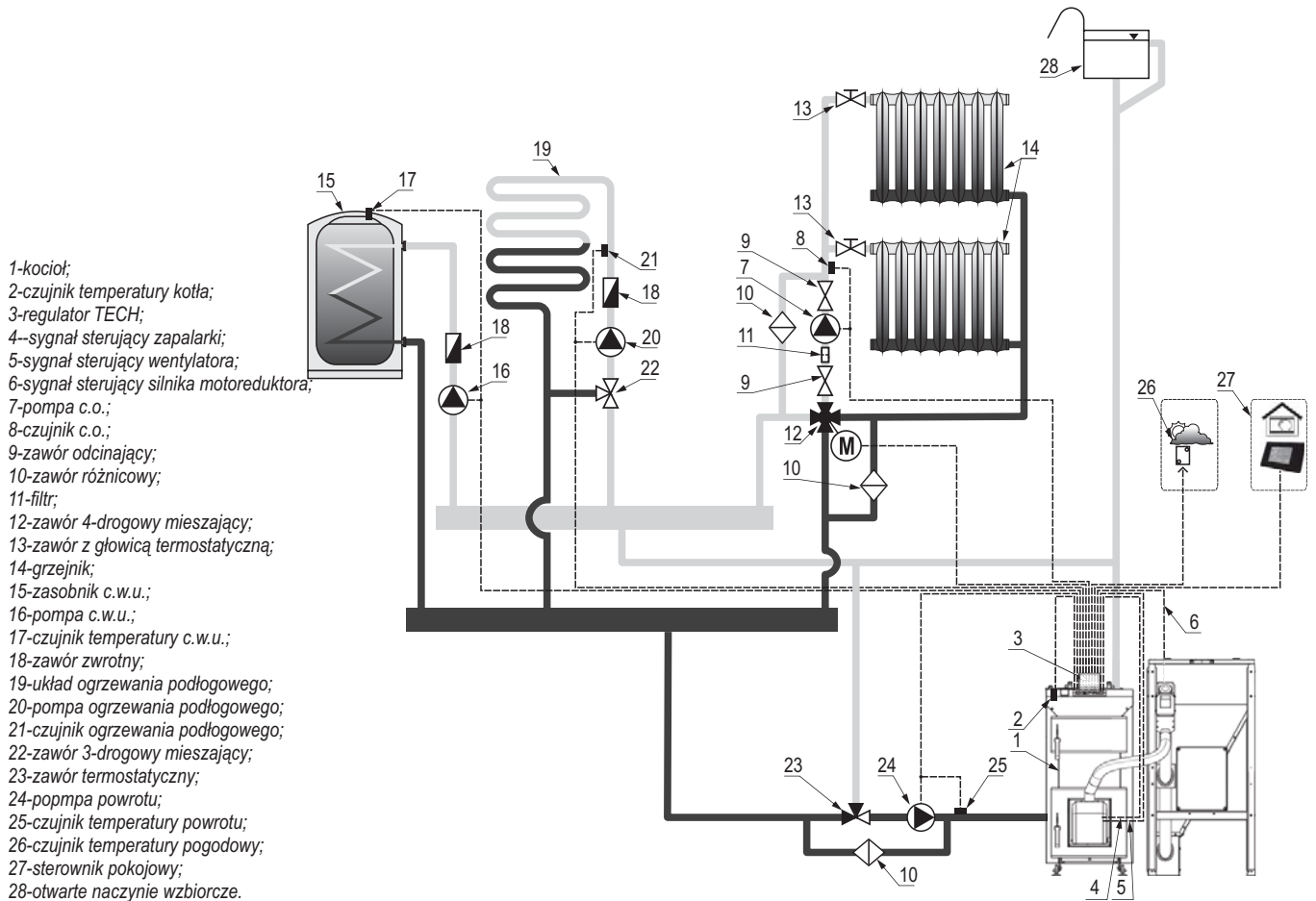
Rysunek 13. Przykładowy schemat instalacji grzewczej systemu otwartego z ochroną temperaturą kotła realizowaną przez zawór termostatyczny.
