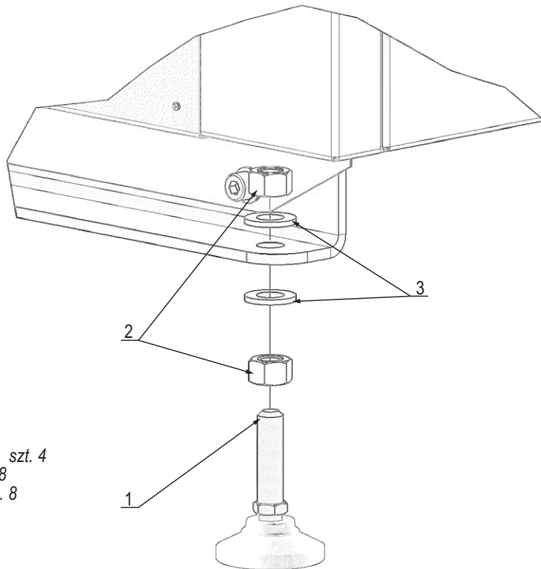
Rysunek 16. Sposób montażu stopek ustalających kocioł.
