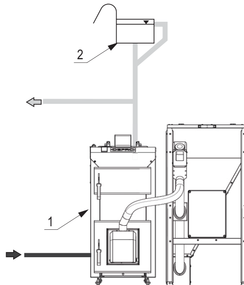
Rysunek 6. Przykładowy schemat zabezpieczeń kotła SIGMA EKOPELL w układzie otwartym: 1-kocioł; 2-otwarte naczynie wzbiorcze.
