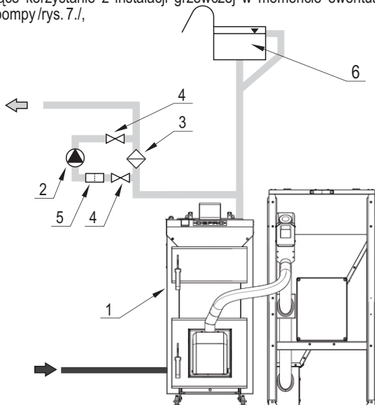
Rysunek 7. Wykonanie obejścia grawitacyjnego: 1-kocioł; 2-pompa obiegowa; 3-zawór różnicowy; 4-zawory odcinające; 5-filtr; 6-otwarte naczynie wzbiorcze.
