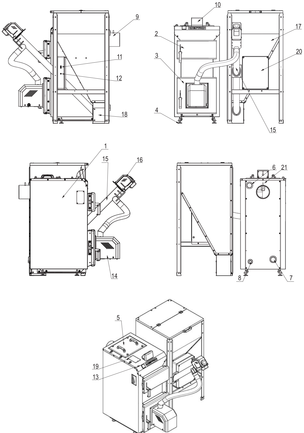
Rysunek 3. Podstawowe elementy kotłów.
