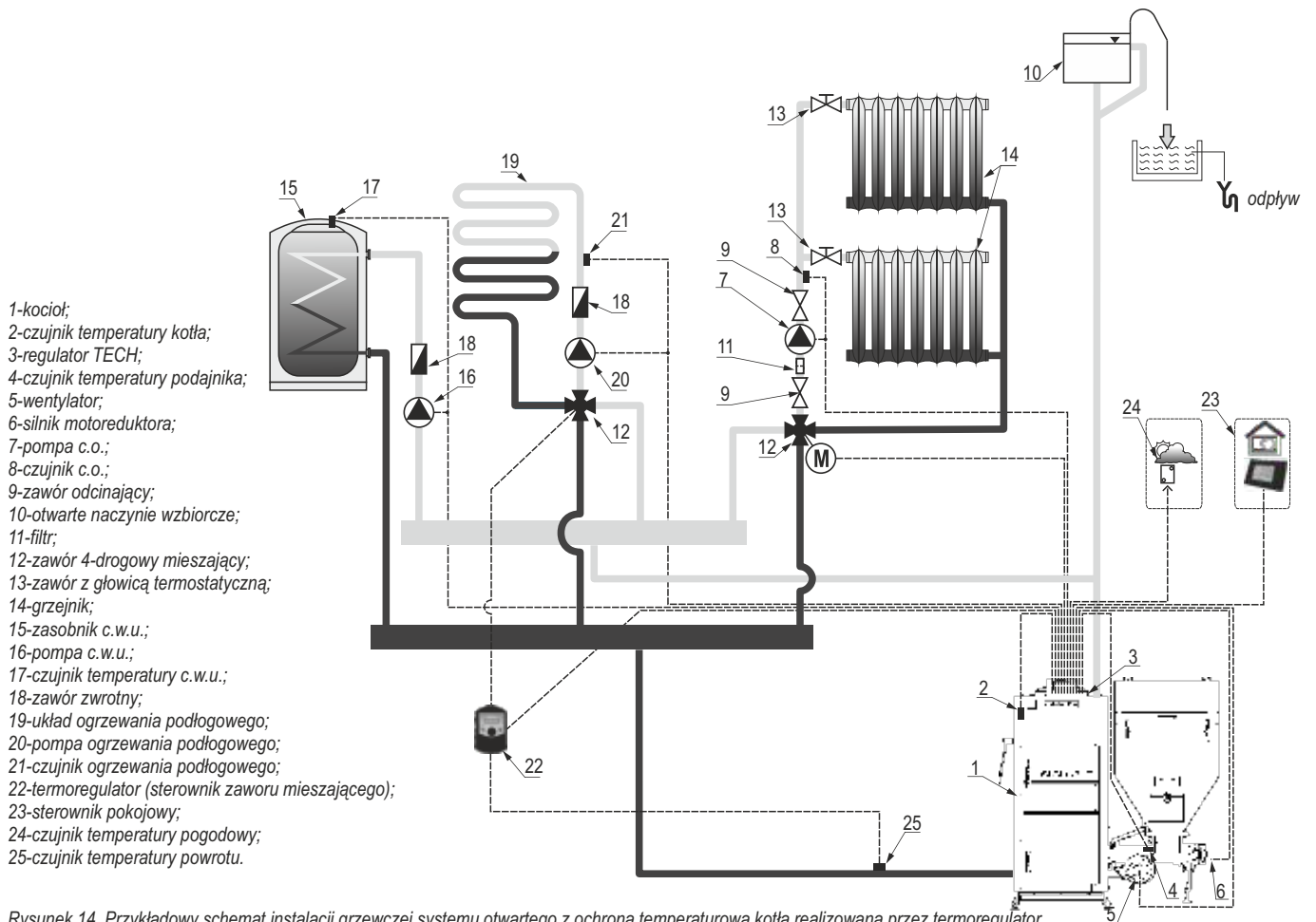
Rysunek 14. Przykładowy schemat instalacji grzewczej systemu otwartego z ochroną temperaturą kotła realizowaną przez termoregulator.
