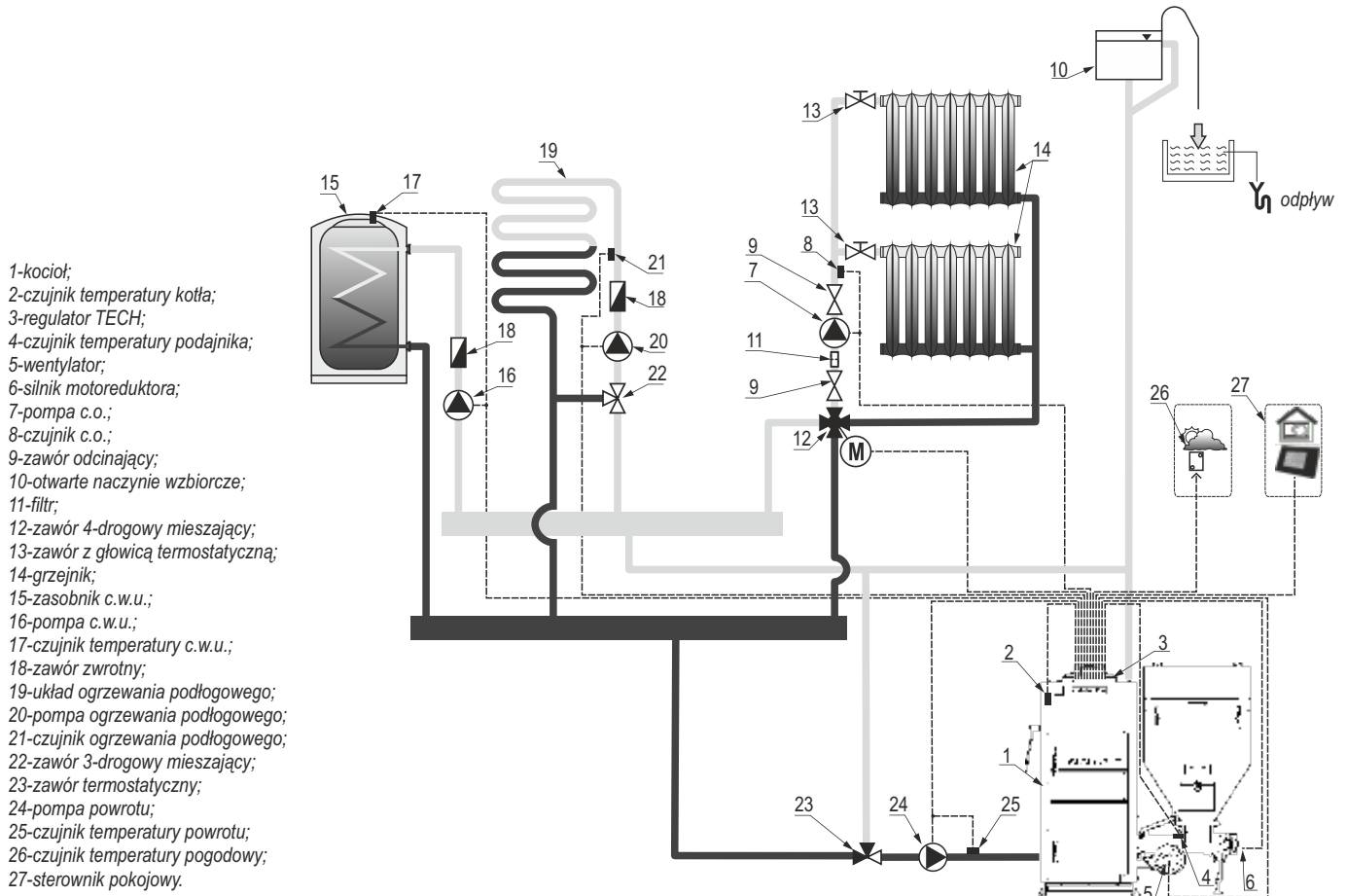
Rysunek 15. Przykładowy schemat instalacji grzewczej systemu otwartego z ochroną temperaturą kotła realizowaną przez zawór termostatyczny.
