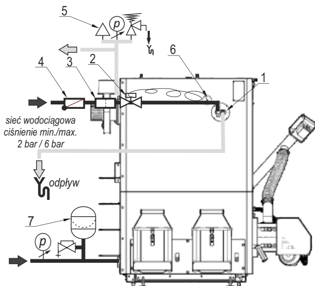
Rysunek 7. Przykładowy schemat zabezpieczeń kotła w układzie zamkniętym: 1-wężywnica; 2-zawór BVTS wkręcony w wężywnicę; 3-filtr wody użytkowej; 4-zawór zwrotny; 5-armatura bezpieczeństwa; 6-czujnik zaworu BVTS; 7- naczynie wzbiorcze przeponowe.
