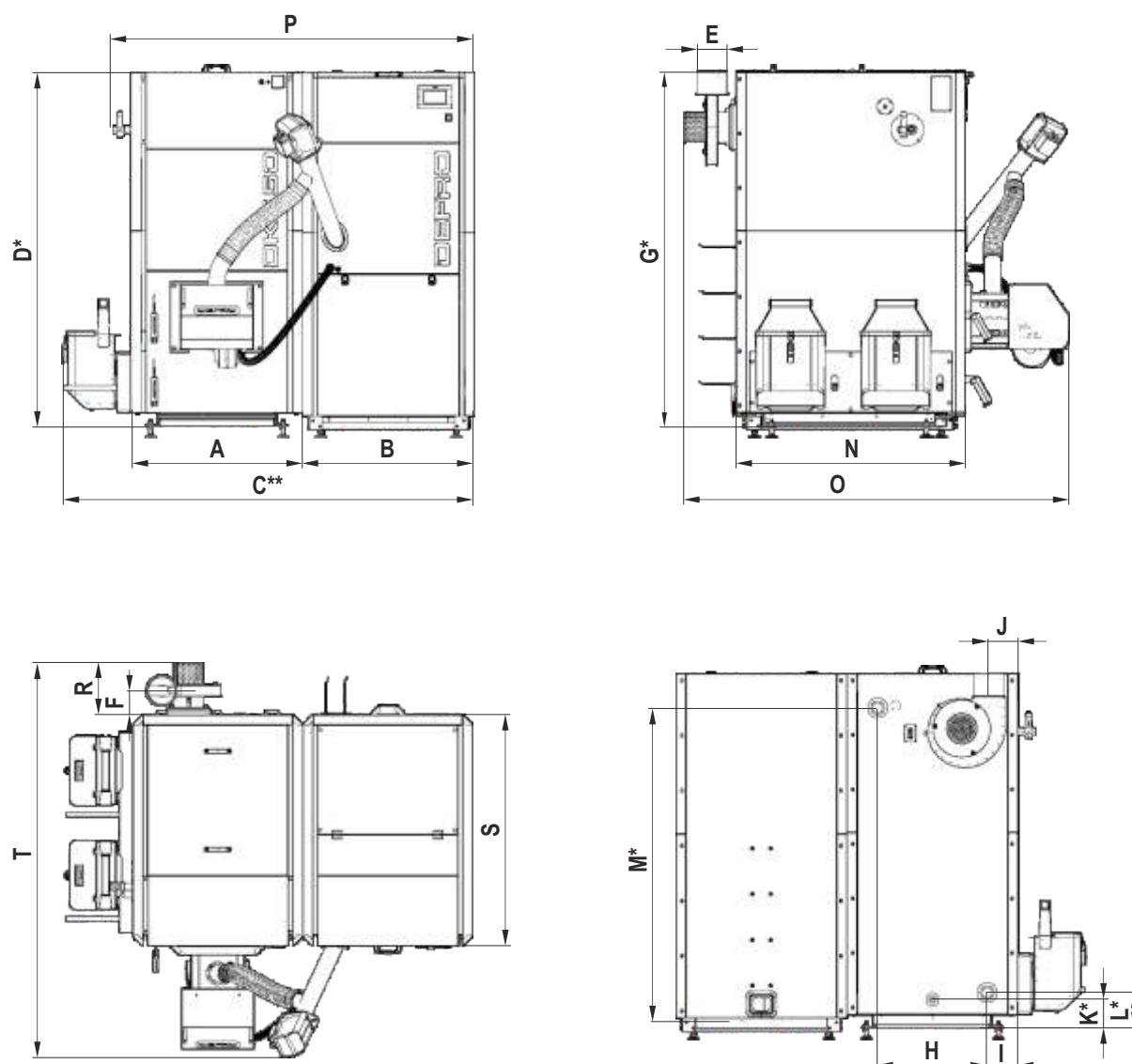
Rysunek 1. Podstawowe wymiary kotłów.
