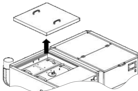
a) zdjąć osłonę pokryw wyczystnej
