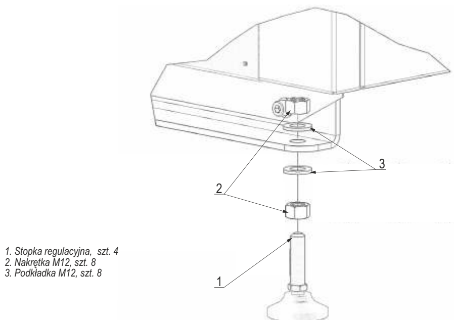
Rysunek 23. Sposób montażu stopek ustalających kocioł.
