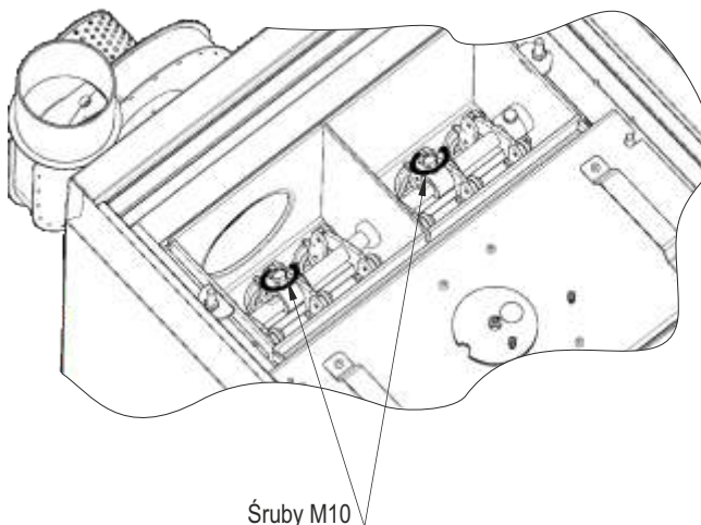
b) usunąć z kotła pokrywę wyczystną
