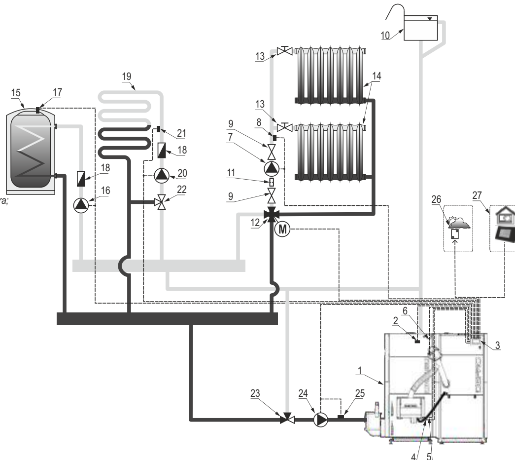
Rysunek 15. Przykładowy schemat instalacji grzewczej systemu otwartego z ochroną temperaturową kotła realizowaną przez zawór termostatyczny.
