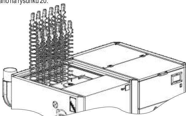
Rysunek 19. Sposób czyszczenia zawirowywaczy.
