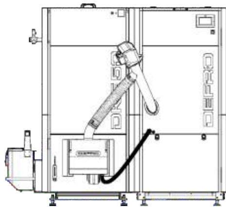
Rysunek 18. Prawidłowe ustawienie zasobnika paliwa względem kotła.
