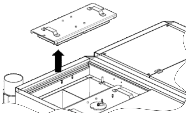
a) zdjąć osłonę pokryw wyczystnej
