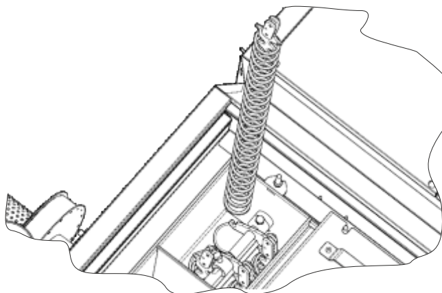
d) ostrożnie wysunąć zawirowywacz z rury płomieniowej, oczyścić; ponowny montaż wykonać w odwrotnej kolejności; sprawdzić poprawność montażu.
