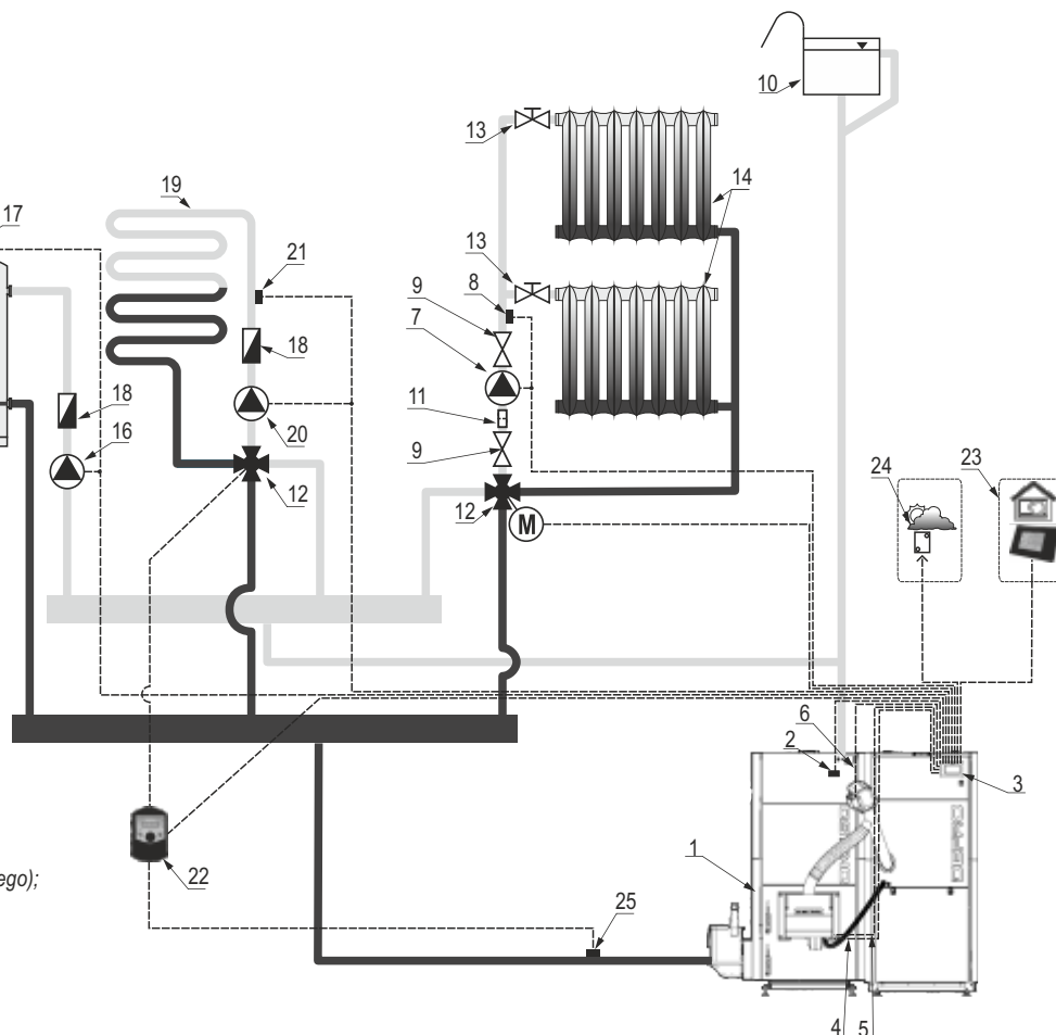
Rysunek 14. Przykładowy schemat instalacji grzewczej systemu otwartego z ochroną temperaturową kotła realizowaną przez termoregulator.
