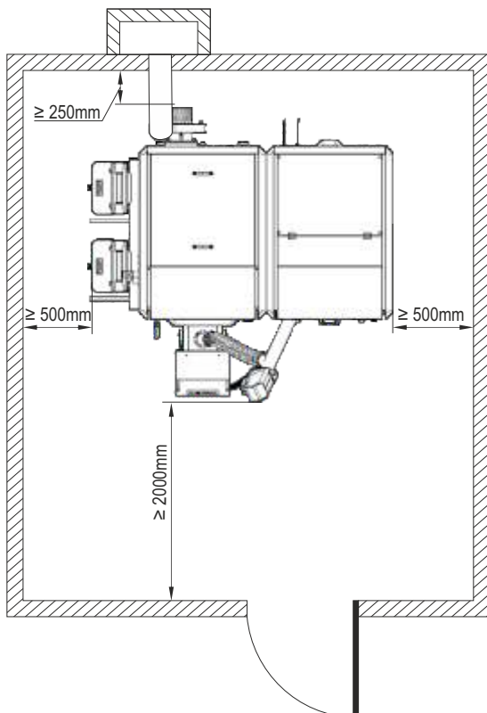
Rysunek 3. Ustawienie kotła w pomieszczeniu kotłowni.
