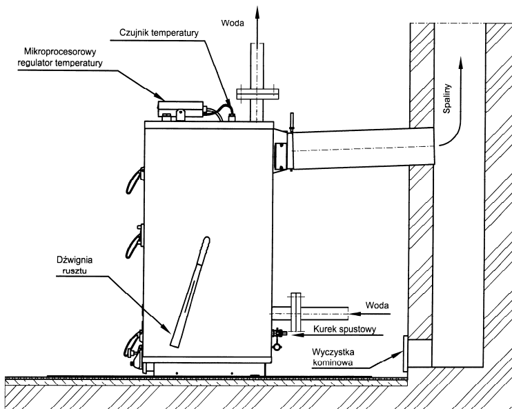
Rys. 1. Przykład podłączenia kotła do instalacji.
